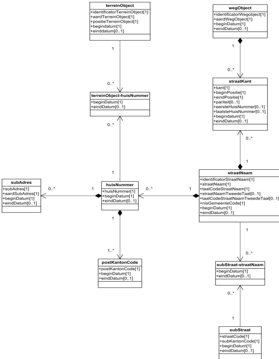
Figuur 1: Conceptueel datamodel
