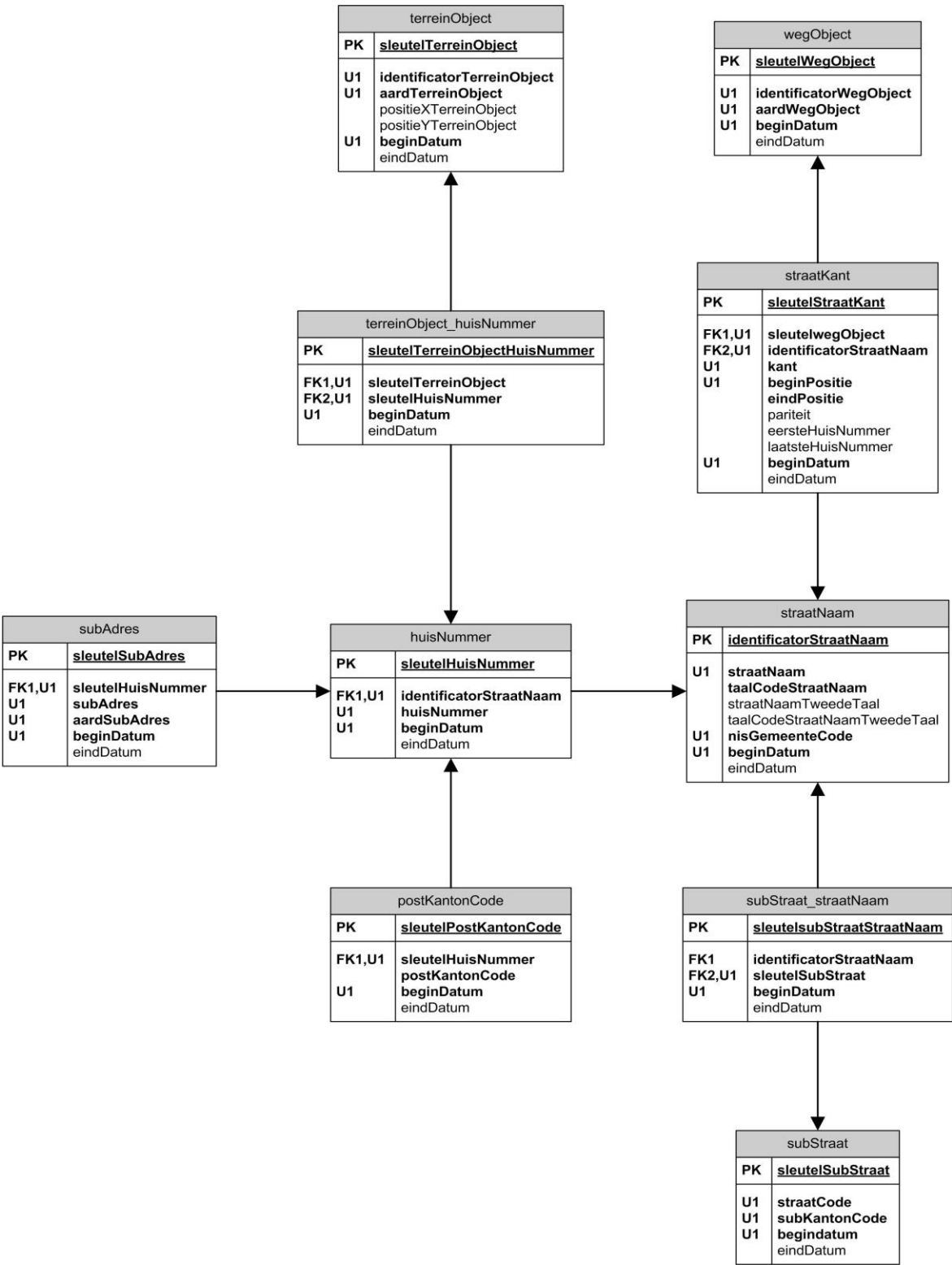
Figuur 2: Logisch datamodel
