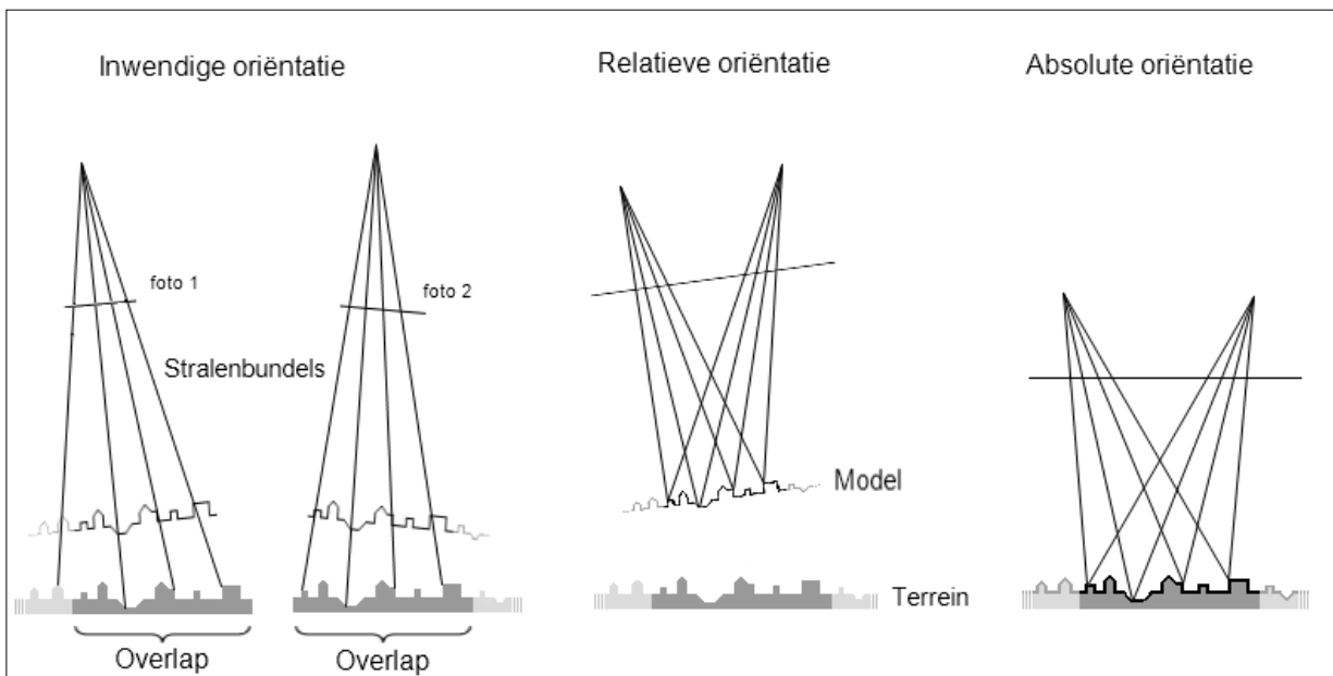
Figuur 1 : opeenvolgende stappen van de aerotriangulatie (inwendige (enkel bij analoge luchtfoto's) en relatieve oriëntatie) en de blokvereffening (de absolute oriëntatie)
